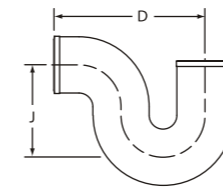
P-Trap
